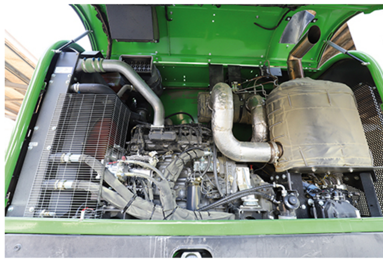
Il motore, un FPT da 260 cavalli, stage 5
